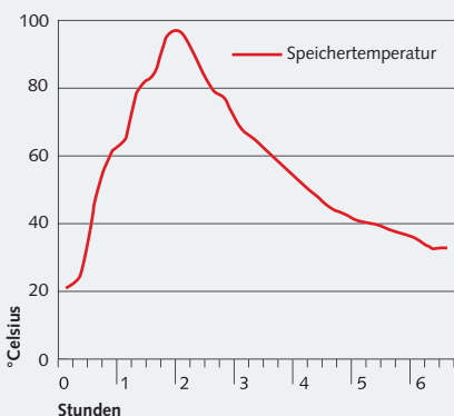
Wärmeabgabe-Diagramm BANDO (Messpunkt: Deckplatte hinten)
